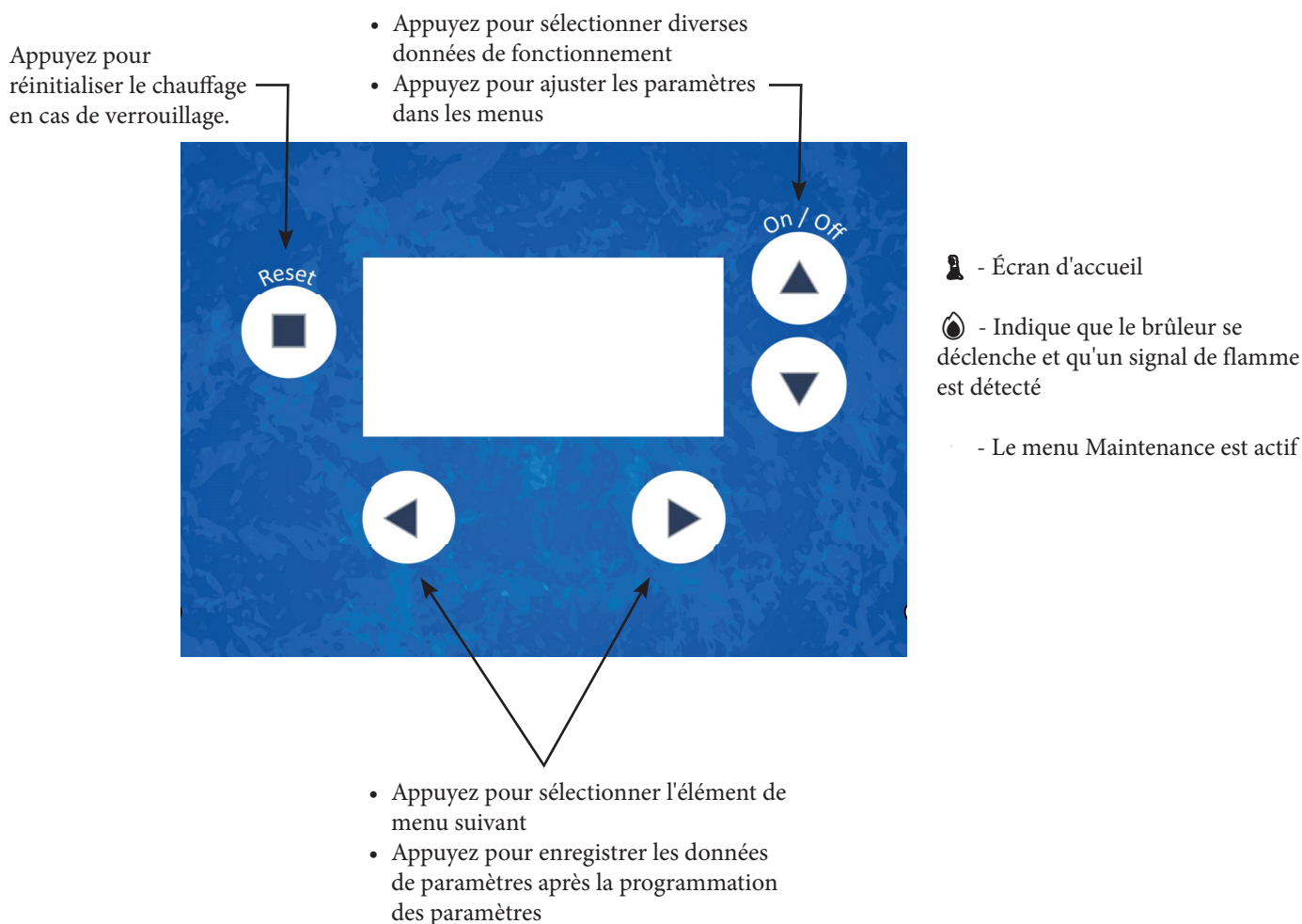
Figure 10-1_panneau de commande
