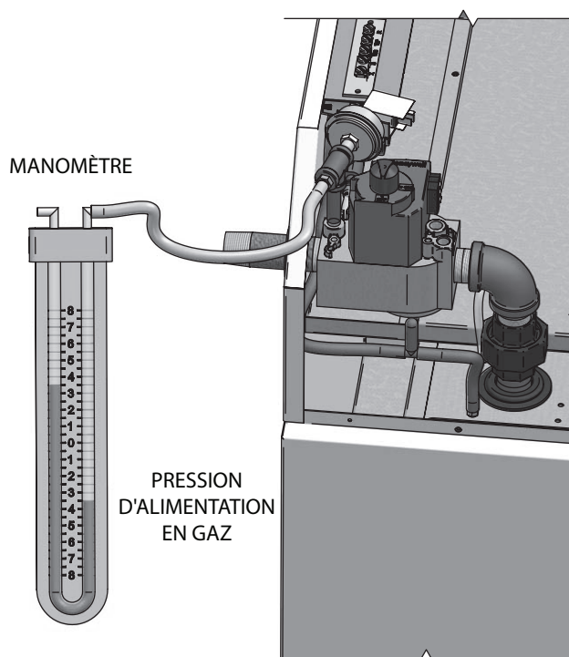
Figure 9-2 Mesure de la pression de gaz d'alimentation - Modèles ER252 - ER402
