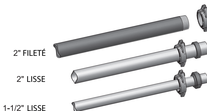
Figure 11-1_ Alternier les raccordements des tuyaux
